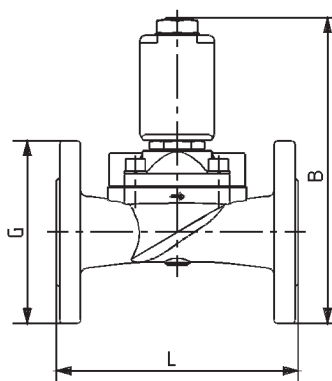
Фланец DIN 2501
